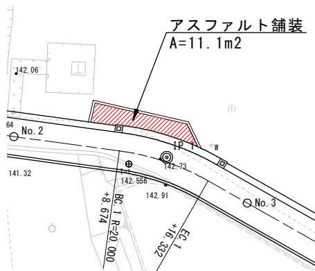
待避所詳細図
